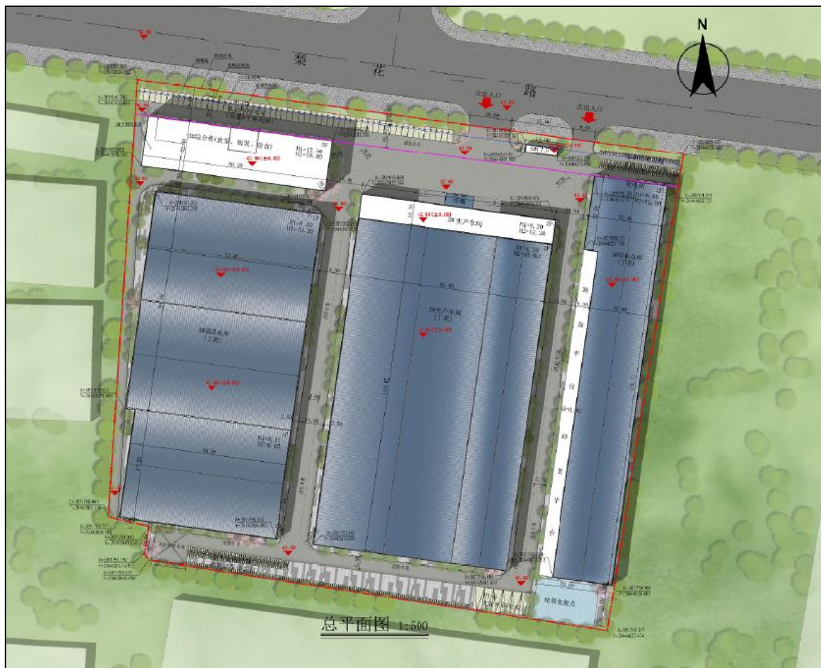
图 1.3 项目总平面布置图
