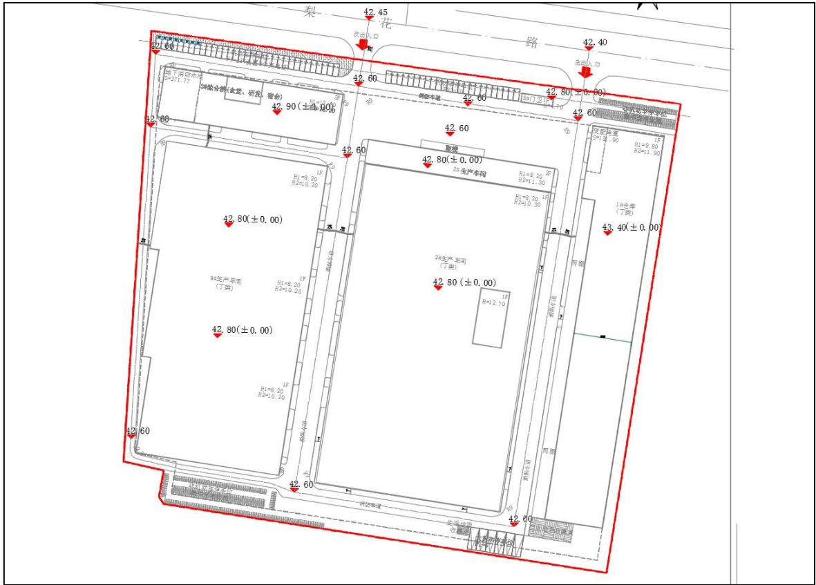
图 1.8 项目竖向布置图
