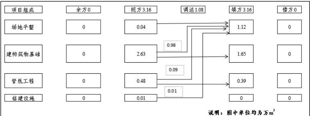
图 1.13 土石方平衡流向框图
