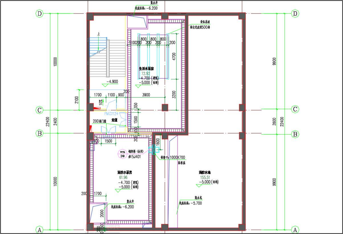
图 1.5 消防水池平面布置图
