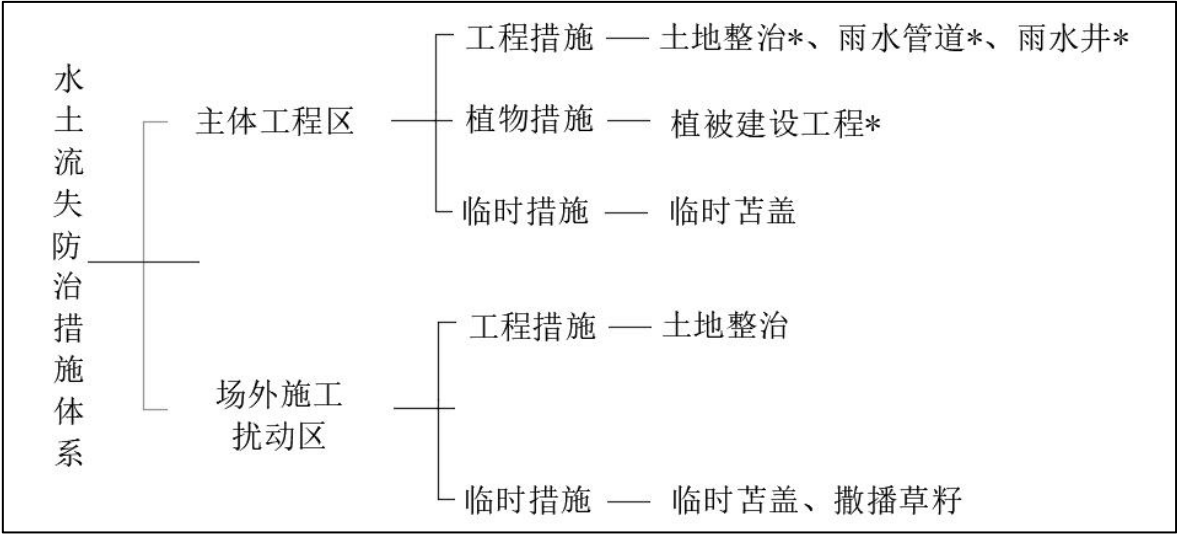
图 5.1 本工程水土流失防治体系框图（带*为主设已列）
