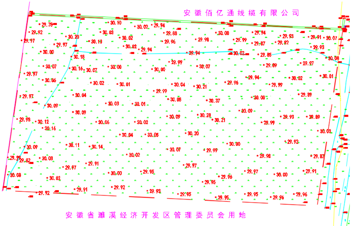
图 1.4 原始标高图
