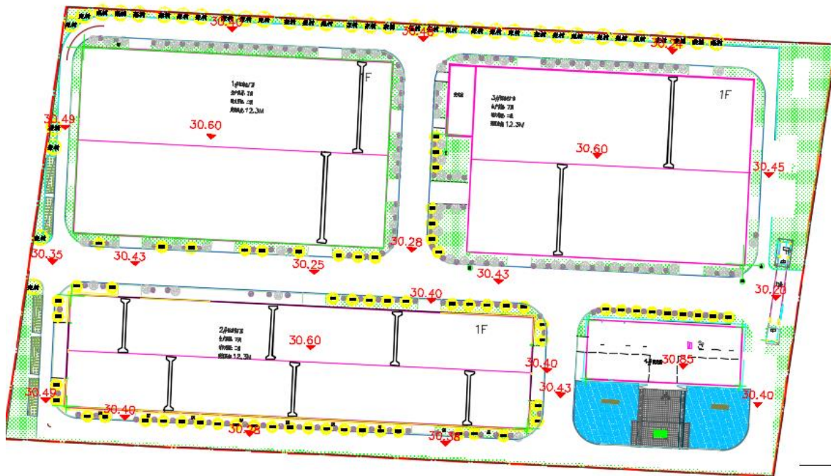
图 1.5 设计标高图
