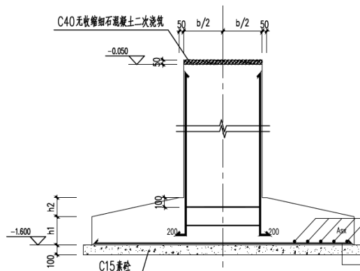
图 1.3 基准桩剖面图
