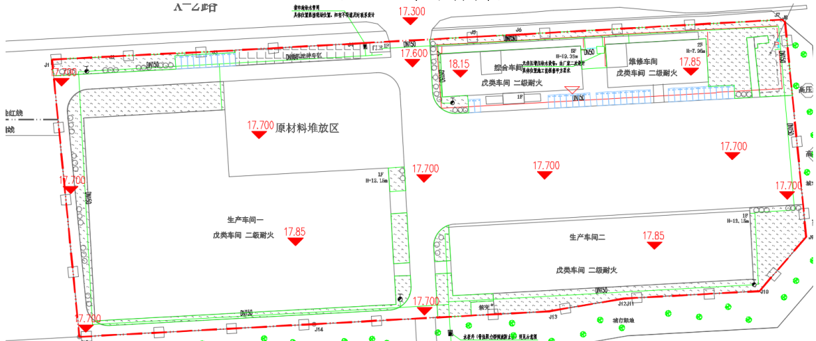
图 1.5 设计标高图
