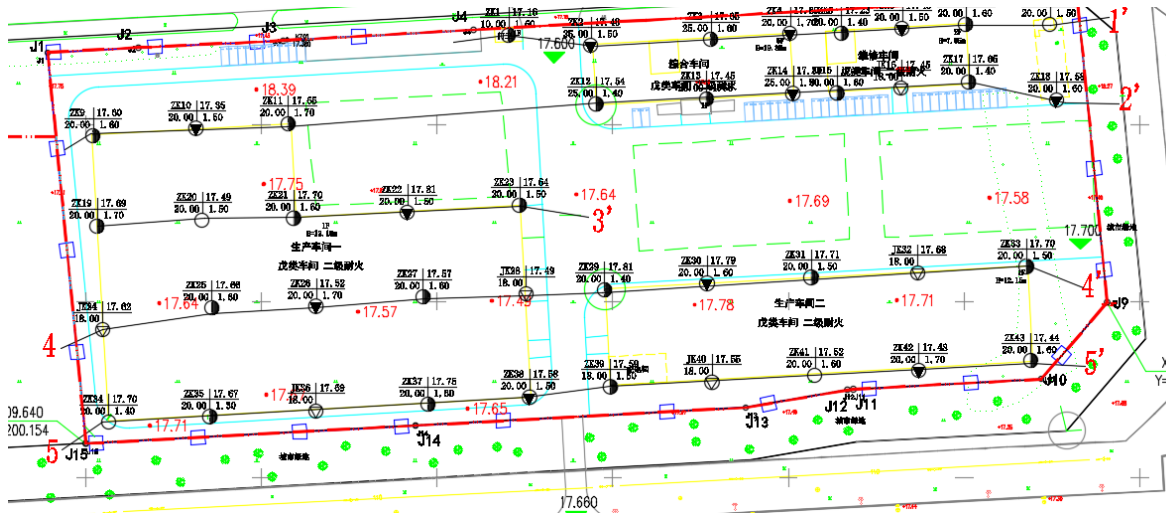
图 1.4 原始标高图
