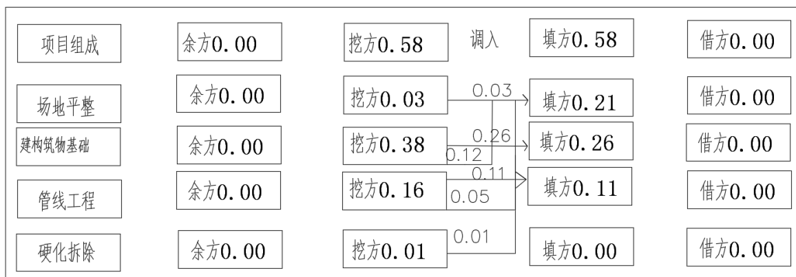
图 1.13 土石方平衡框图
