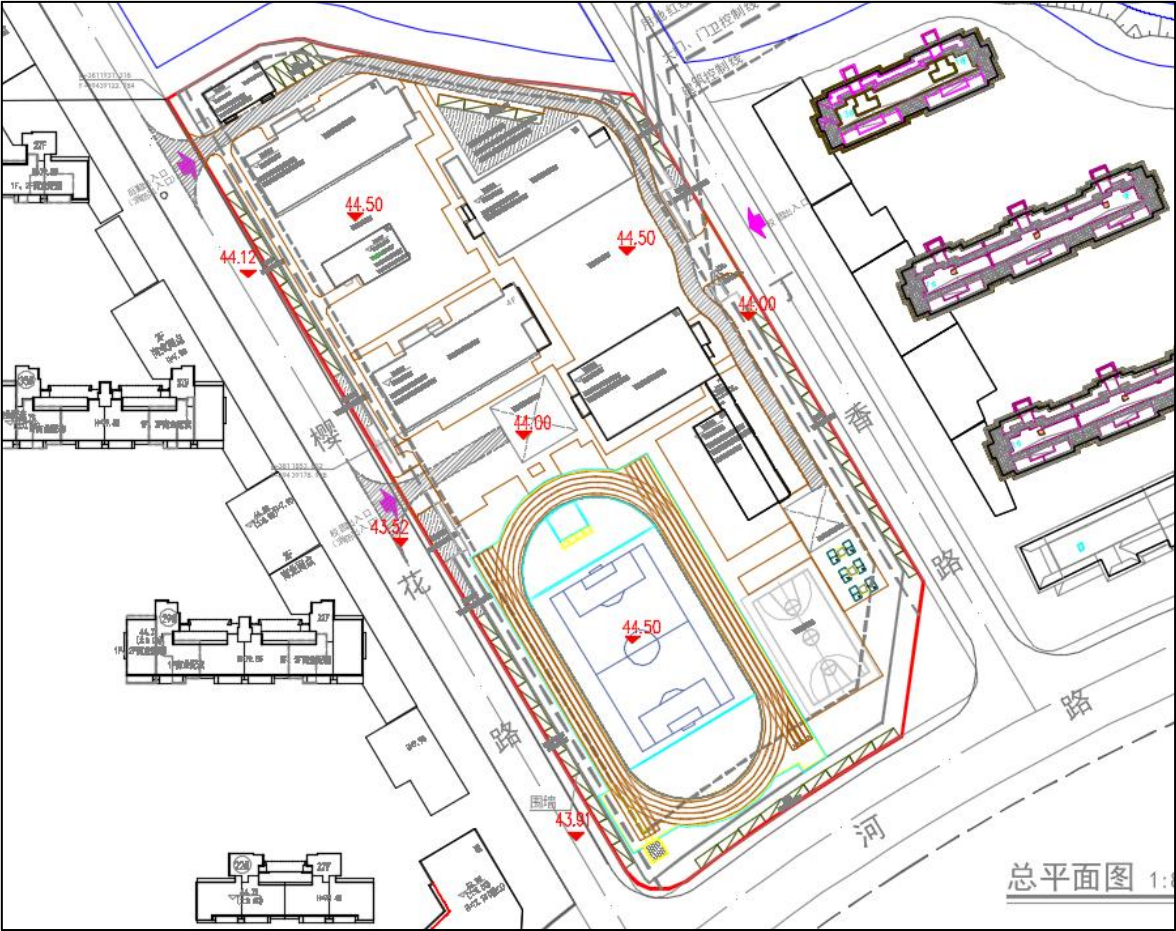
图 1.5 项目竖向布置图
