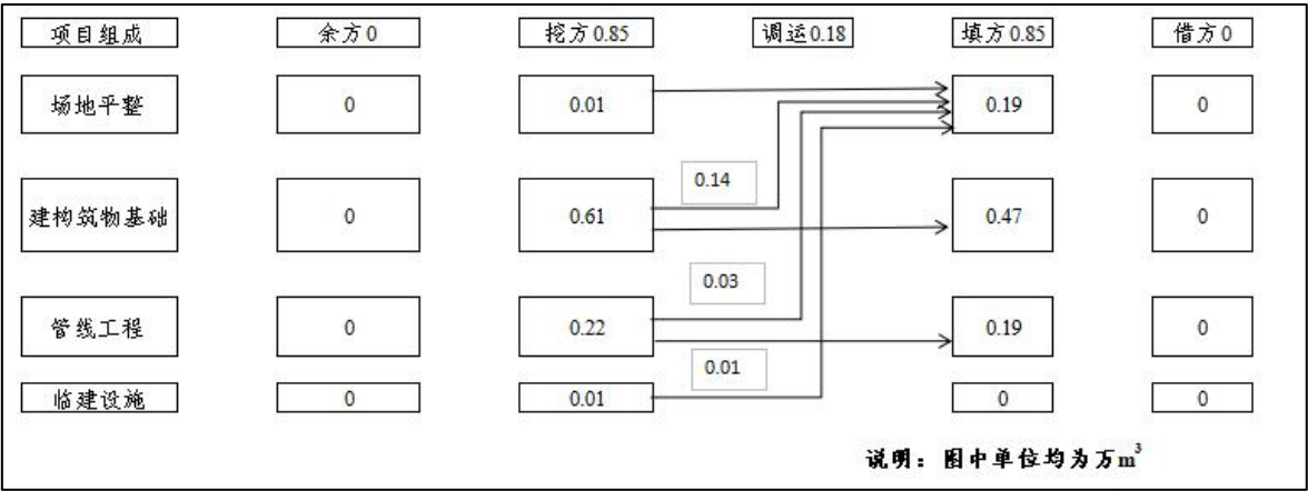
图 1.10 土石方平衡流向框图
