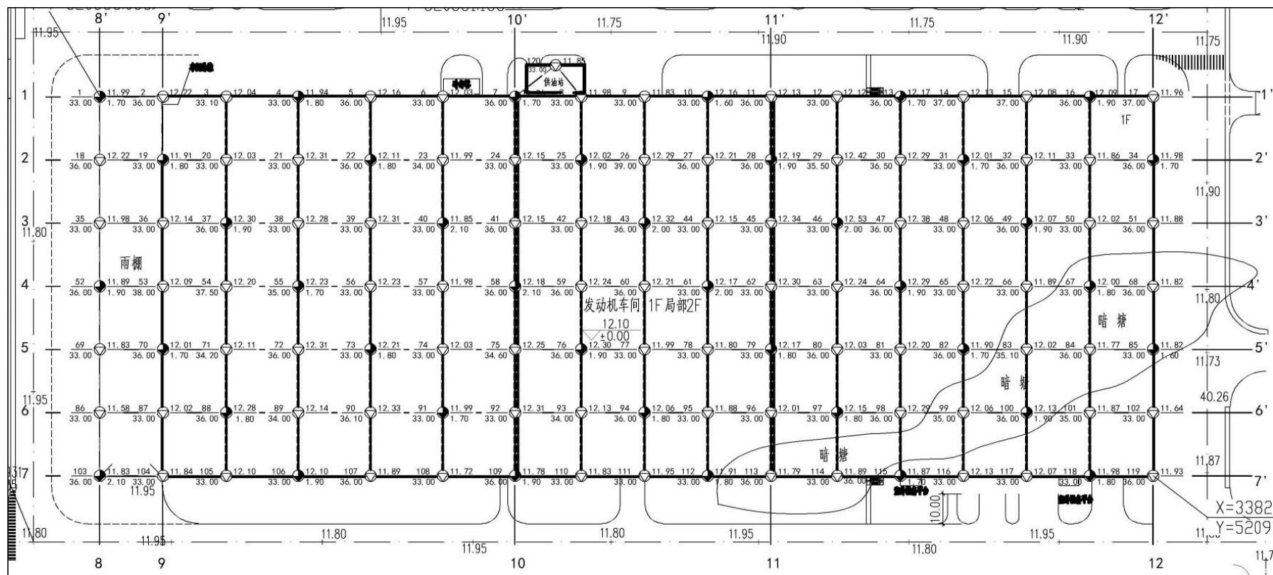
图 1.2-2 项目原地貌标高
