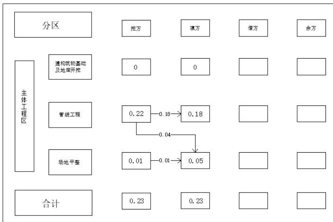
图 1.5-3 待实施土石方平衡 单位：万 m³
