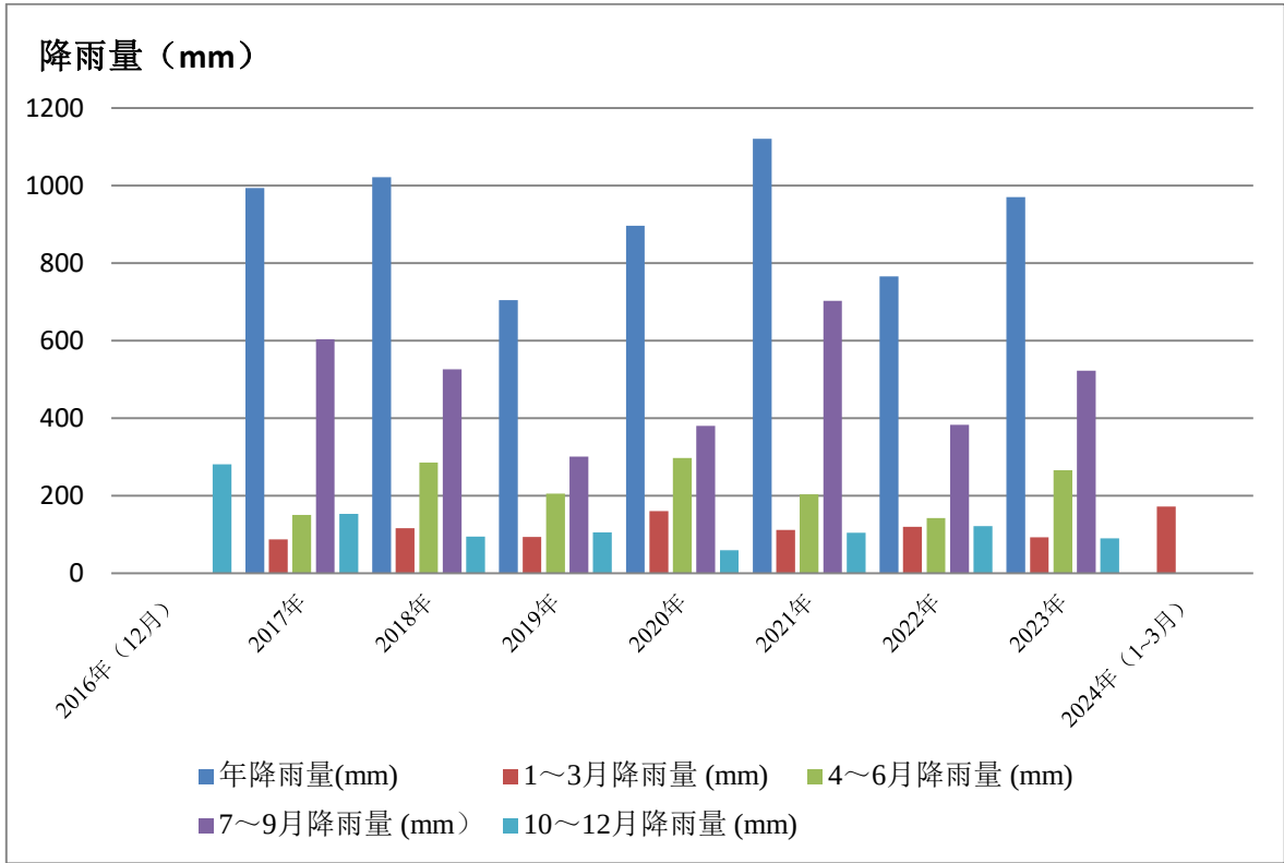
图 5.2 项目降雨量柱状图
