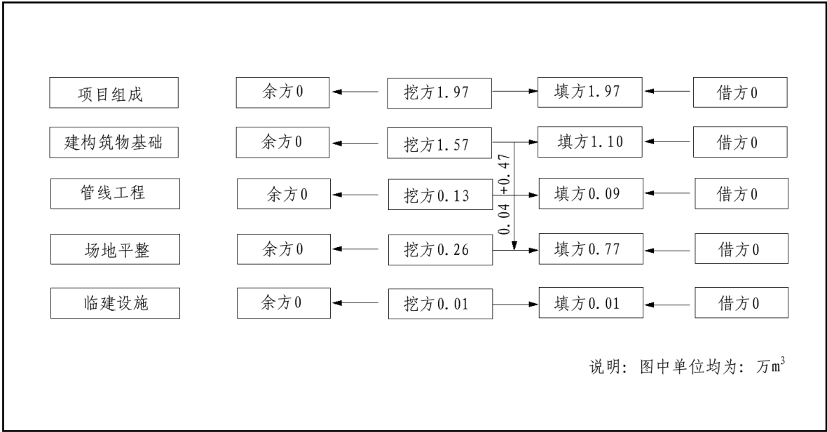
图 1.8 土石方平衡框图
