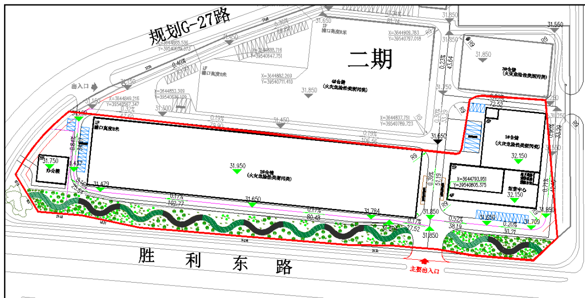
图 1.2 项目总平面图
