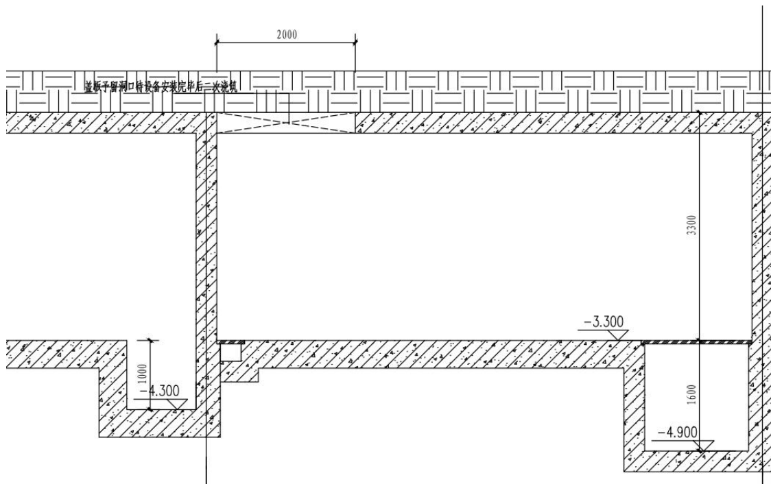
图 1.2-2 地下消防水池/泵站竖向布置图
