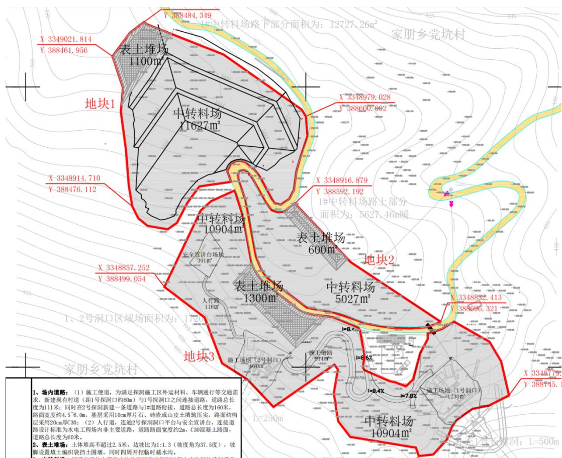
图 1.2-1 项目总体布置图
