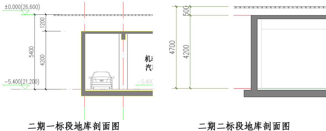
图 1.3 地库剖面图
